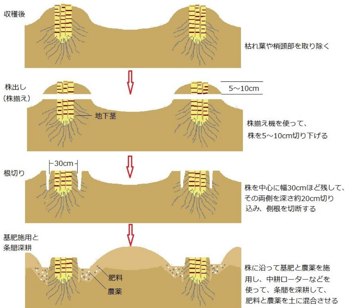
図 5. サトウキビの株出しと根切り模式図
